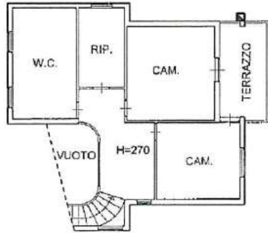
PIANO PRIMO
