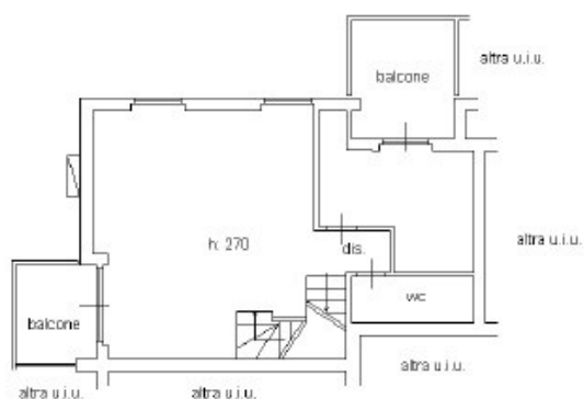
PIANO PRIMO
